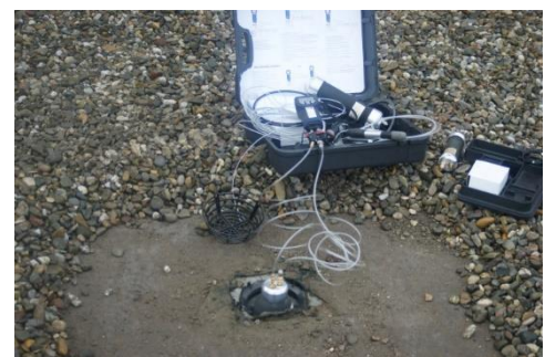
Bild 3: Dichtigkeitsprobe bei Dachentwässerungen
